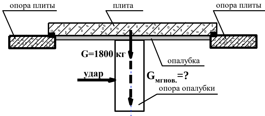
Рисунок 13 – Раскружаливание в строительстве
