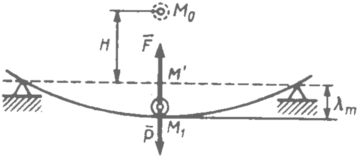
Рисунок 12 – Падение тела на упругую балку
