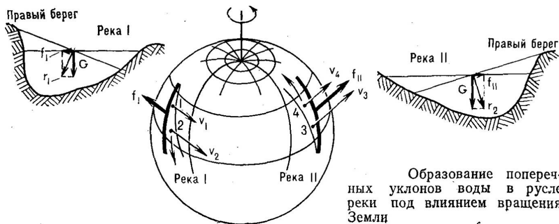
Рисунок 6 – Поперечные уклоны реки
