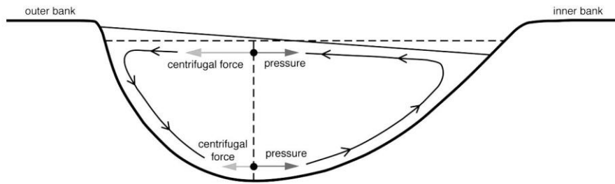
Рисунок 7 – Поперечное закручивание воды в русле реки
