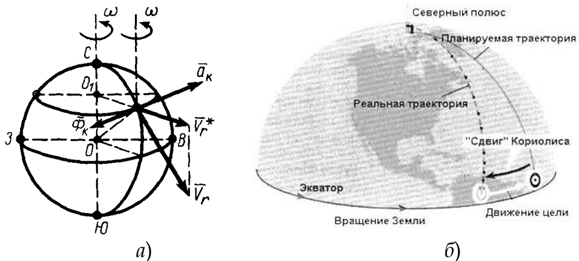
Рисунок 1 – Ускорение и сила инерции Кориолиса
