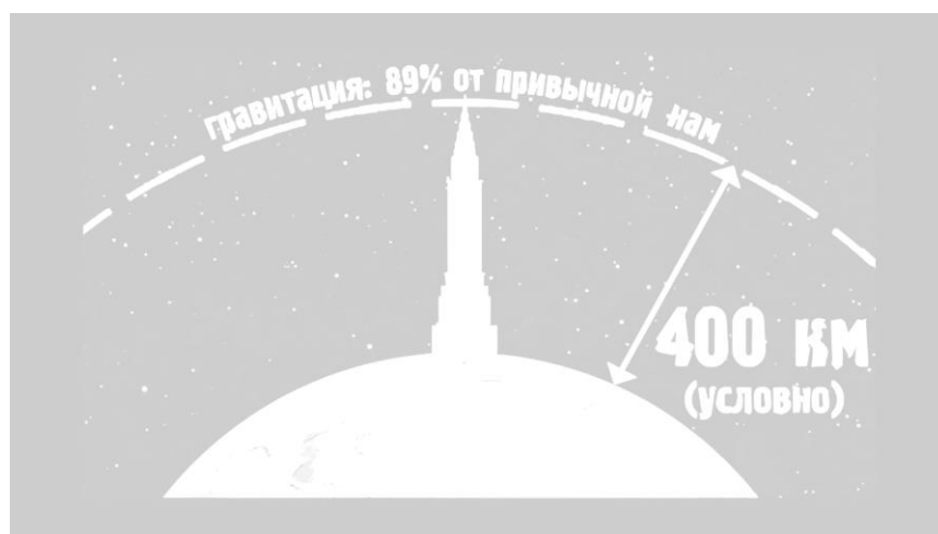
Рисунок 23 – Траектория спутников и МКС
